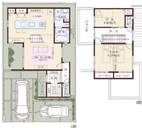
間取り図
